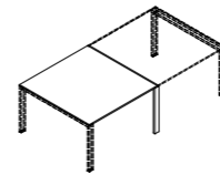
D1212 120x120x74h D1412 140x120x74h D1612 160x120x74h D1812 180x120x74h D2012 200x120x74h D2212 220x120x74h tavolo allineato P120 aligned table D120
