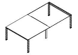
D1414 140x140x74h D1614 160x140x74h D1814 180x140x74h D2014 200x140x74h D2214 220x140x74h tavolo allineato P140 aligned table D140
