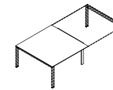
SQD1414 140x140x74h SQD1614 160x140x74h SQD1814 180x140x74h SQD2014 200x140x74h SQD2214 220x140x74h tavolo allineato P140 aligned table D140
